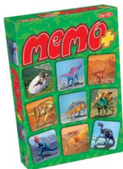
MEMO+ dinosaurier 01725
