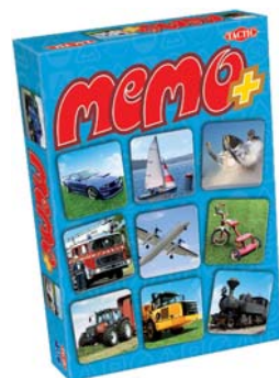
MEMO+ fordon 01724
